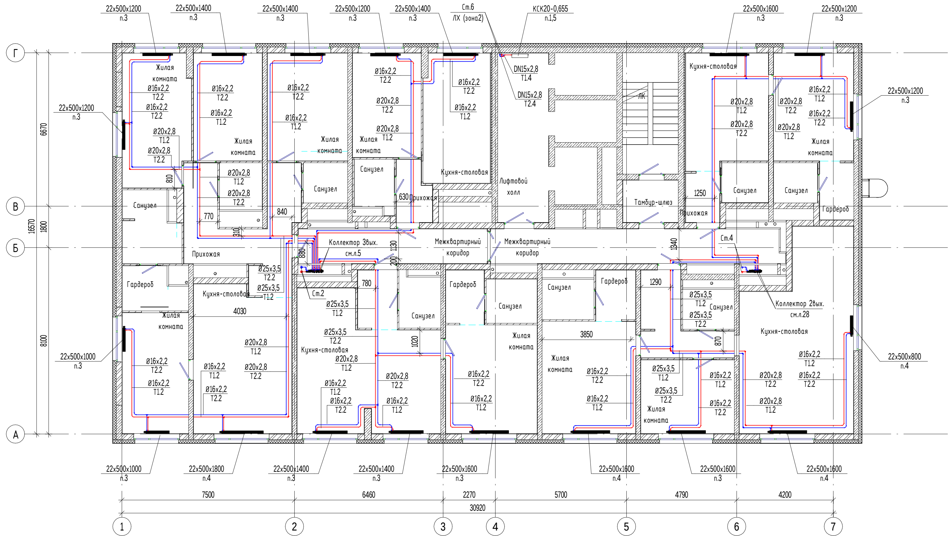
Коллектор на 8 выходов (16-24 этаж, Ст.4)
