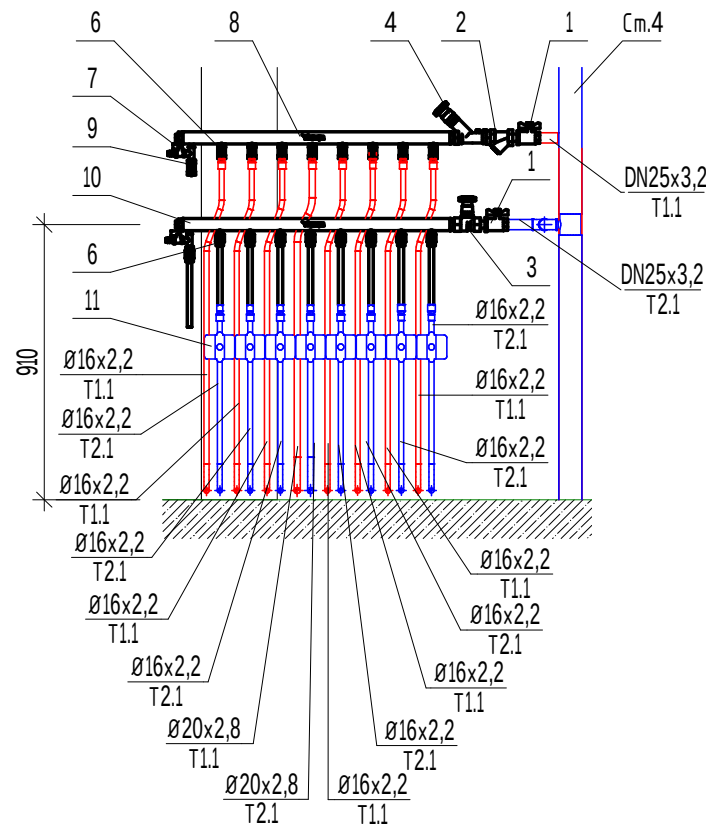
Коллектор на 8 выходов (16-24 этаж, Ст.4)
